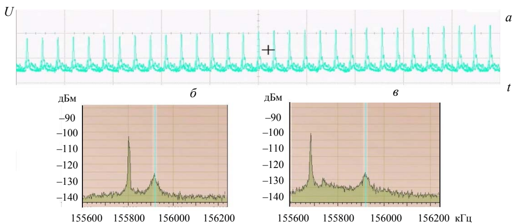
Рис. 2. Осциллограмма напряжения с фотодиода (а), t = 20 нс/дел, U = 20 мВ/дел, и радиоспектры (б) и (в); разность длин волн 0.3 (а, б) и 0.4 нм (в)
